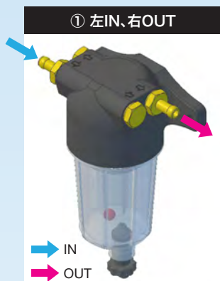
左方から右方に流れる管路
